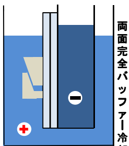
泳動槽断面図
