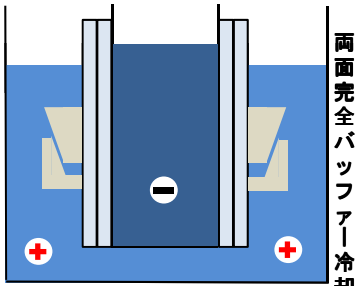
泳動槽断面図
