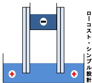
泳動槽断面図
