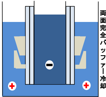
泳動槽断面図
