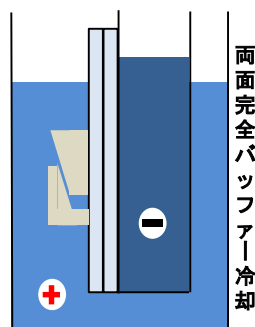
泳動槽断面図
